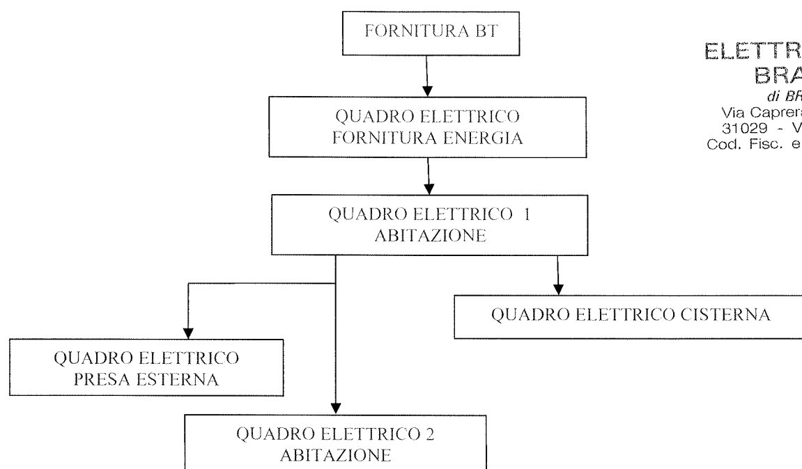
Schema a blocchi distribuzione Q.E.
