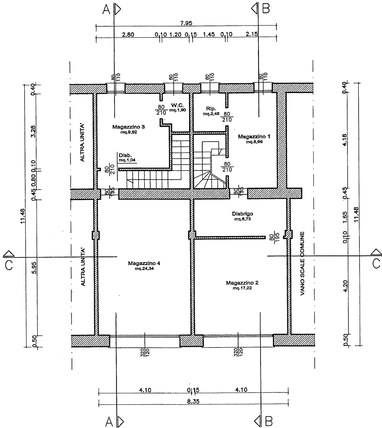
Piano Primo scala 1:100
